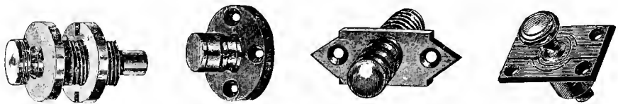
Fig. 4469. END-DOOR-SASH BOLT.
